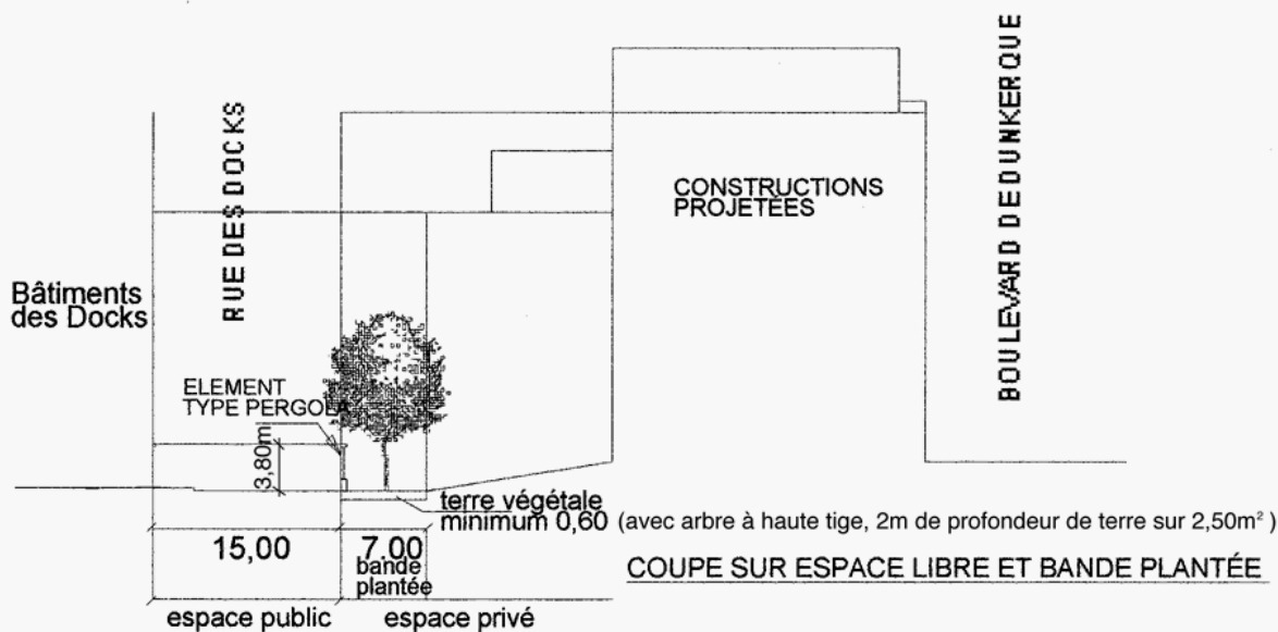
COUPE SUR CONSTRUCTIONS PROJÉTÉES À L'ALIGNEMENT
